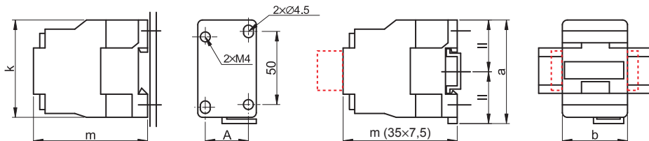
Mocowanie do płyty montażowej
