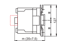
Mocowanie na szynie montażowej (35x7,5 mm)
