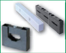
Nośniki szyn i ich osłony (rozstaw osi szyn: 60 mm) 18
